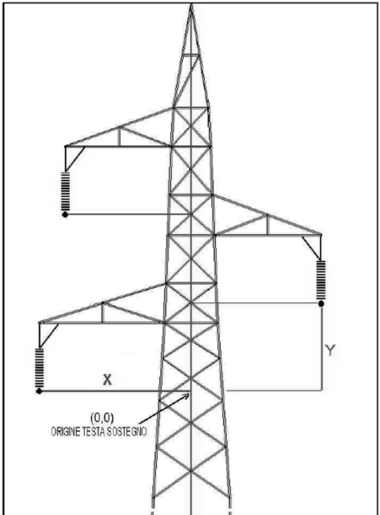
Sistema di riferimento del sostegno
